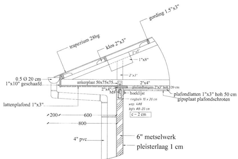
detail kap Schaal 1 : 20
