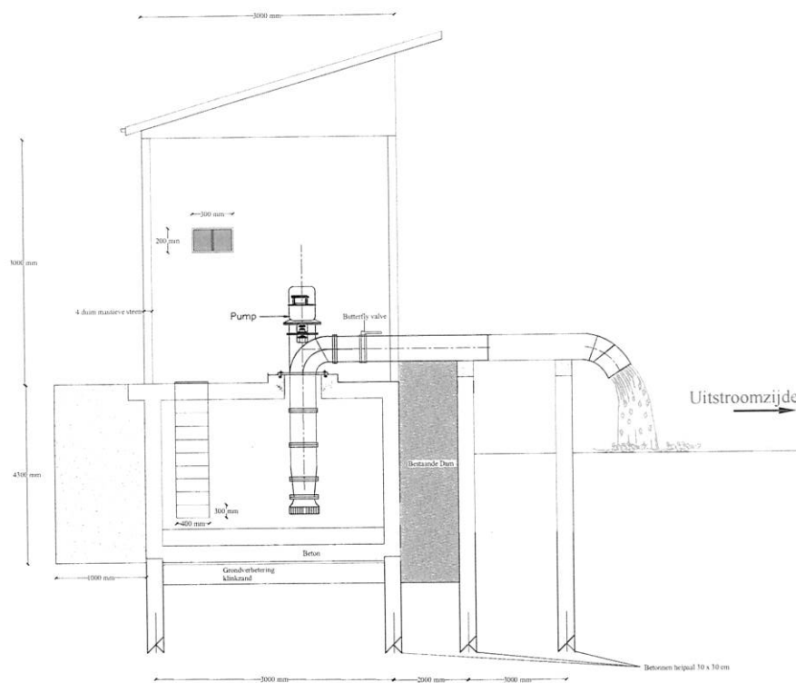
ZIJ-AANZICHT
