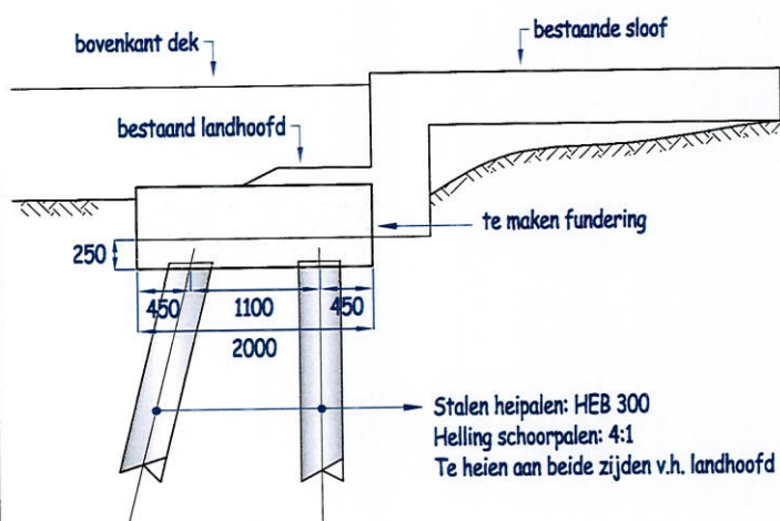
ZIJTAAZNICHT LANDHOOFD
