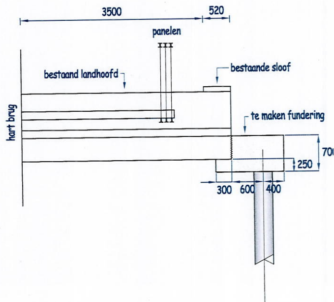
VOORAANZICHT LANDHOOFD
