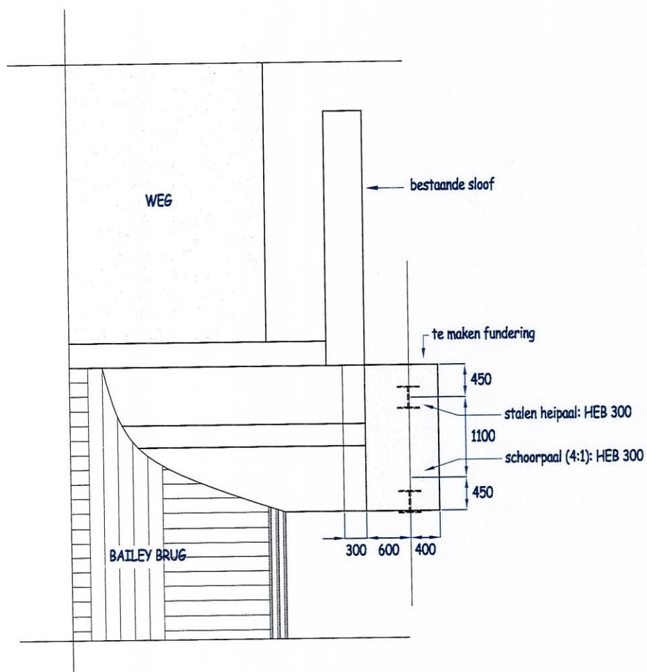
BOVENAANZICHT LANDHOOFD
