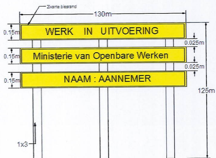
VOOR AANZICHT
