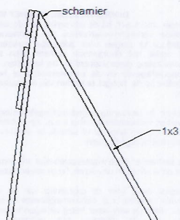
ZIJ AANZICHT
