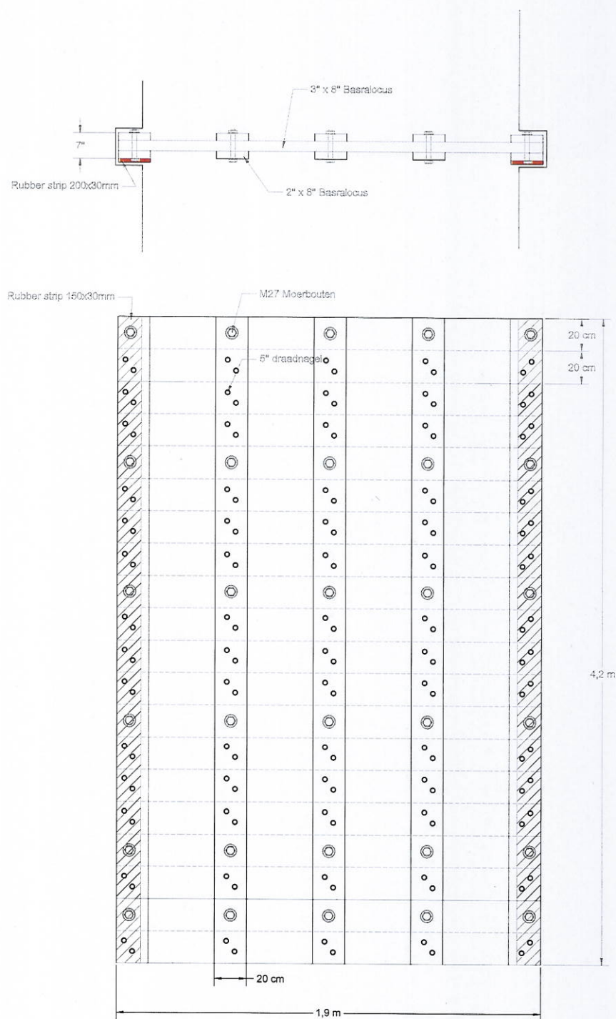
Principe houten sluisdeur Koendanlal
