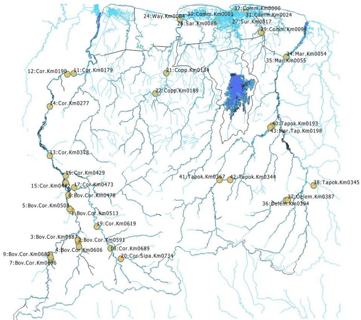
Figuur 44: Virtueel observatie station : Data worden via satelliet om de 27 dagen geregistreerd.
