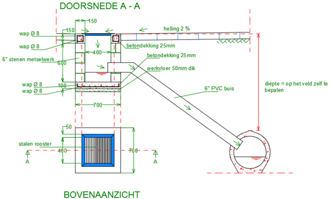
Schema 2: Perceelaansluiting
