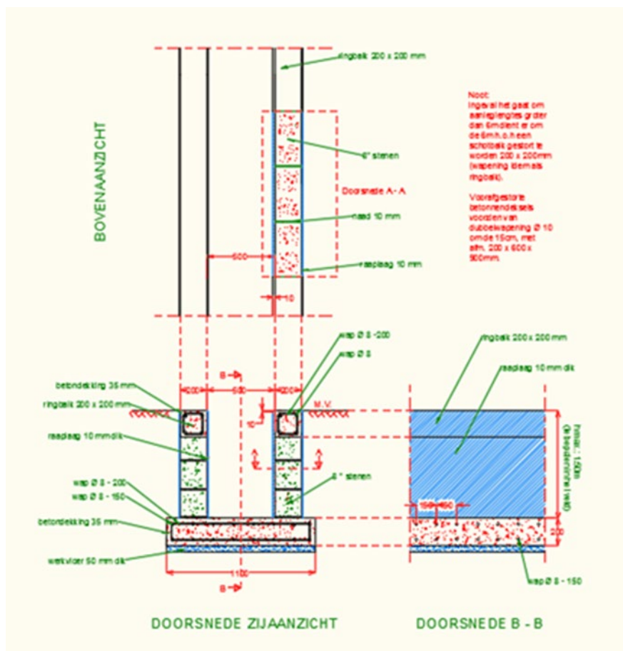
Schema 1: Eenvoudige duikerconstructie
