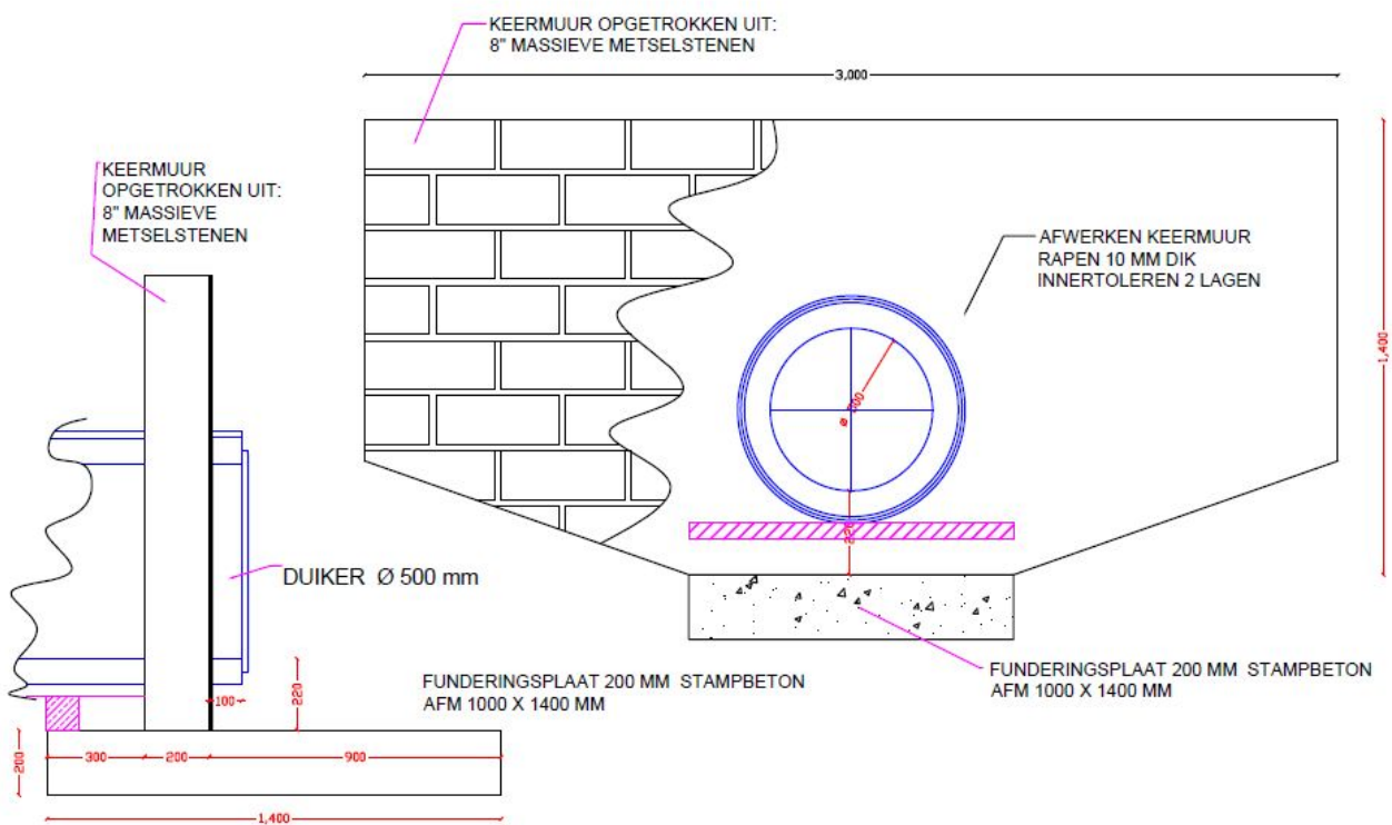
Schema 3: Eenvoudige keermuur
